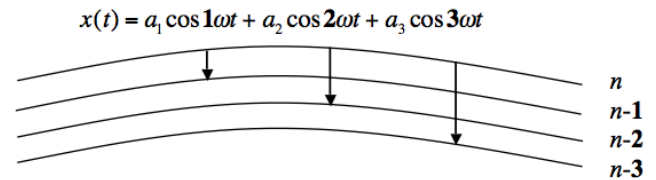
Figur 2. En klassisk baneurve opløst i Fourierkomponenter [2]. Ifølge korrespondensprincippet svarer enhver tilladt overgang mellem stationære baner til en af den klassiske bevægelses harmoniske komponenter.
